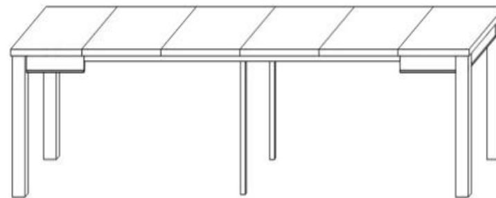
A30 R Stół po rozłożeniu 2900 / 750 / 902
