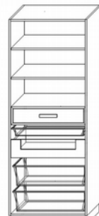
Segment 13 Szer. 600-900 mm wys. 2100-2400 mm gł. 600 mm
