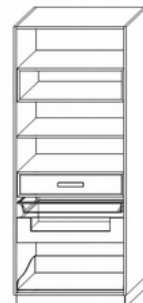
Segment 11 Szer. 600-900 mm wys. 2100-2400 mm gł. 600 mm
