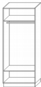
Segment 2 Szer. 400-1000 mm wys. 2100-2400 mm gł. 400-600 mm
