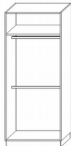
Segment 3 Szer. 400-1000 mm wys. 2100-2400 mm gł. 400-600 mm
