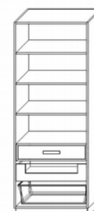
Segment 14 Szer. 600-900 mm wys. 2100-2400 mm gł. 600 mm
